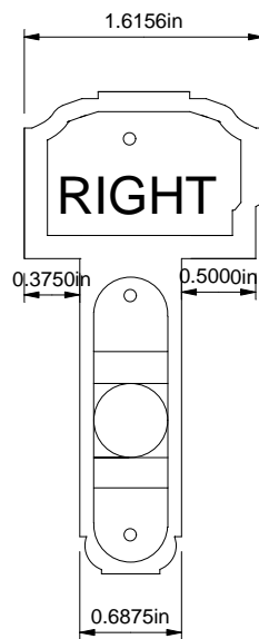
T-astragal Boot - RH
